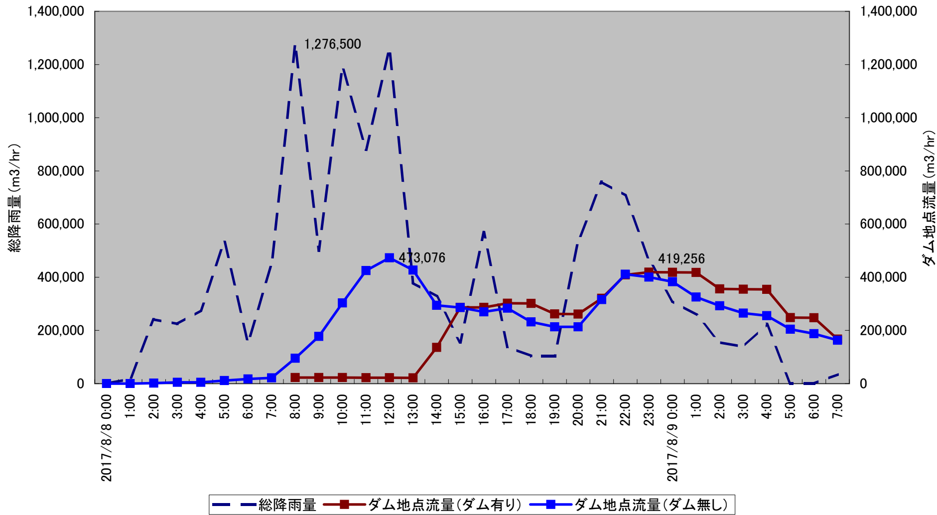
内川ダム 総降雨量とダム地点流量(ダム有り・無し)
