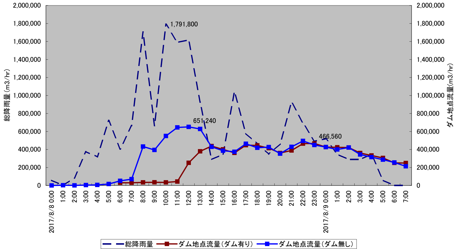
犀川ダム 総降雨量とダム地点流量(ダム有り・無し)
